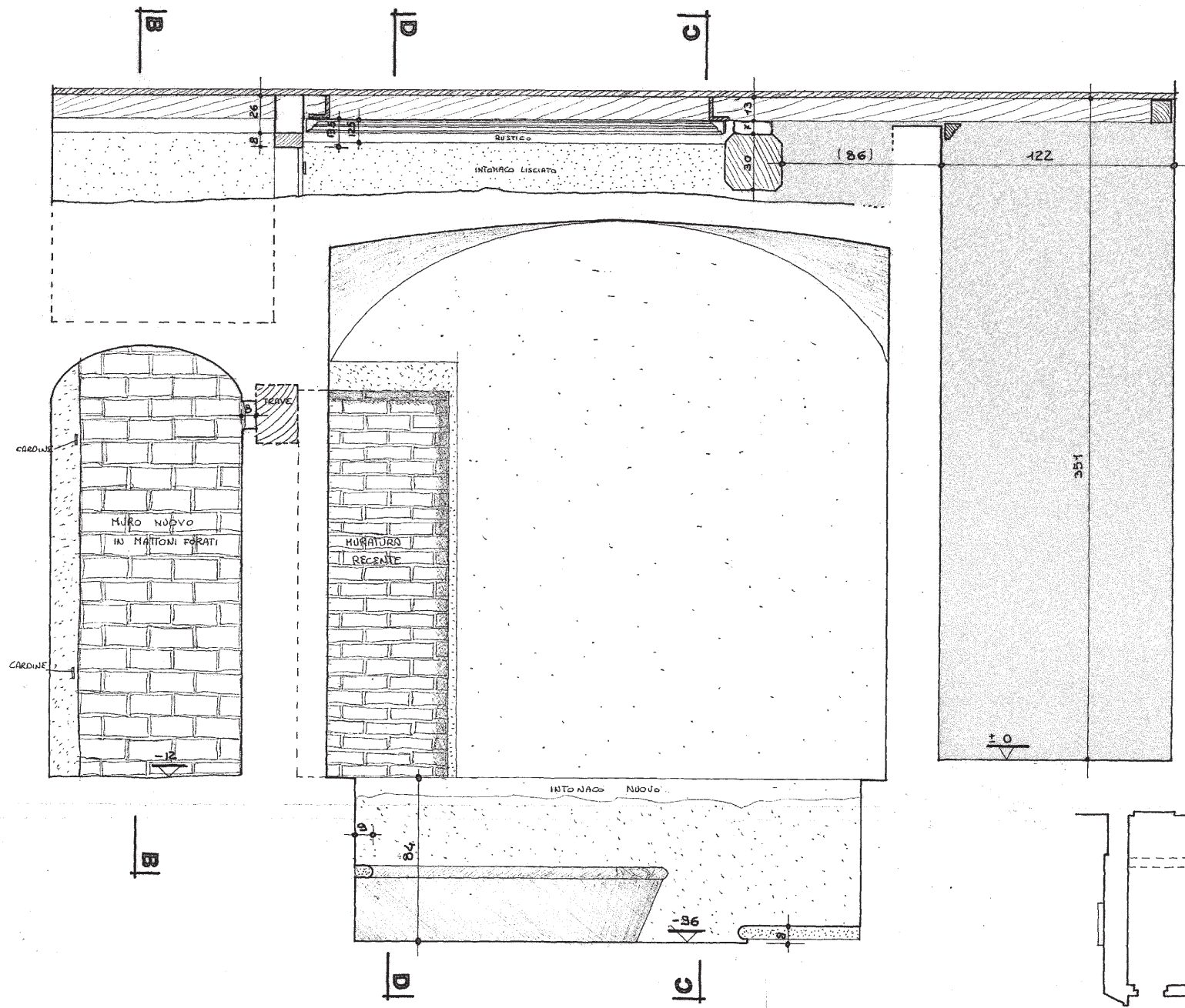
SEZIONE EE VEDERE ANCHE LE SEZIONI BB CC DD
