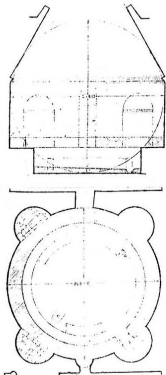
Pompei, Terme Stabiane, pianta e sezione del Laconicum da: Eschembach
