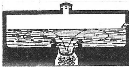
Schema di funzionamento del riscaldamento della acqua nei bagni Turchi (grandi impianti)
