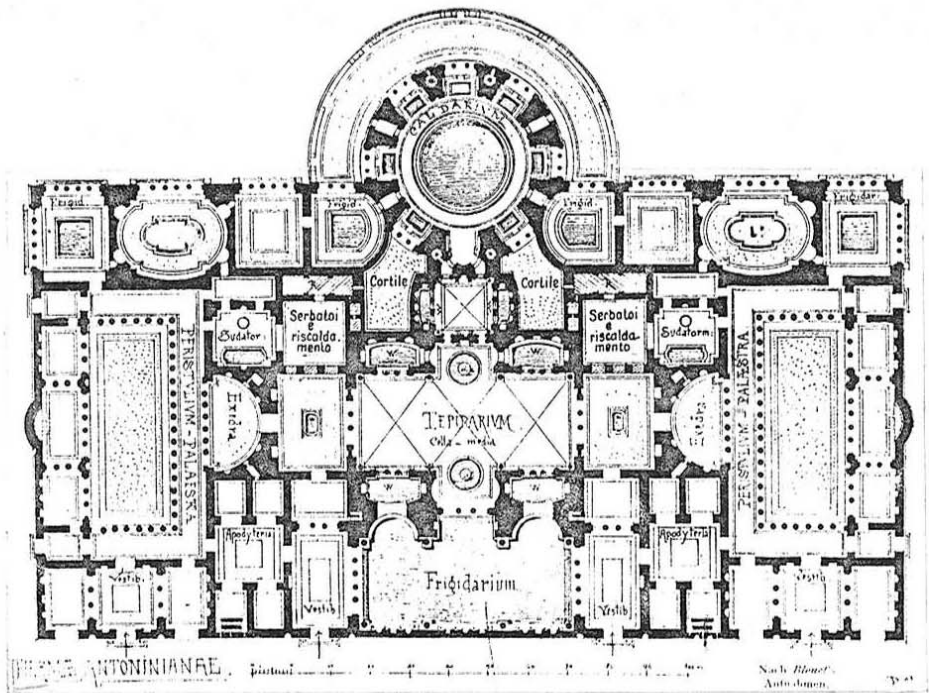
Roma, Terme di Caracalla, ricostruzione; da: Durm
